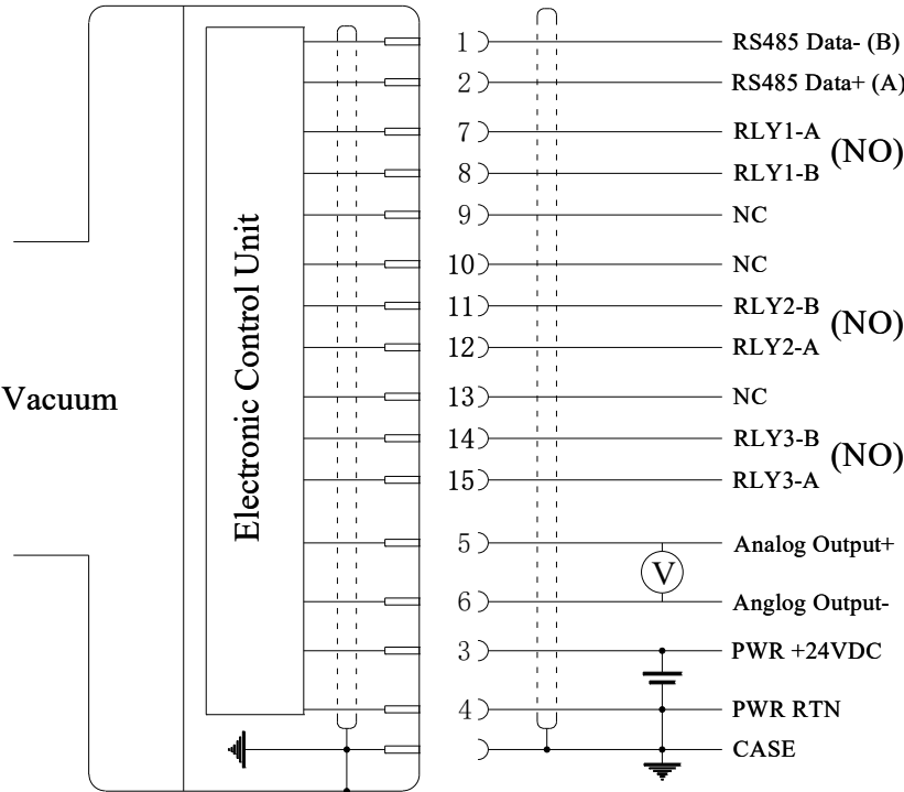
真空计D-Sub 15 VGA功能图
